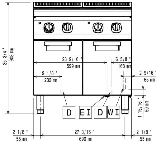
Oldalnézet
